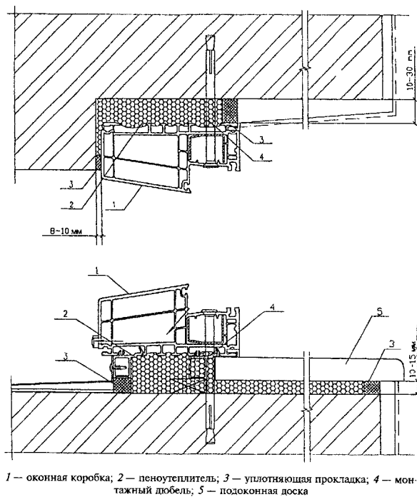
Рисунок Г.1 — Пример монтажного узла оконного блока
