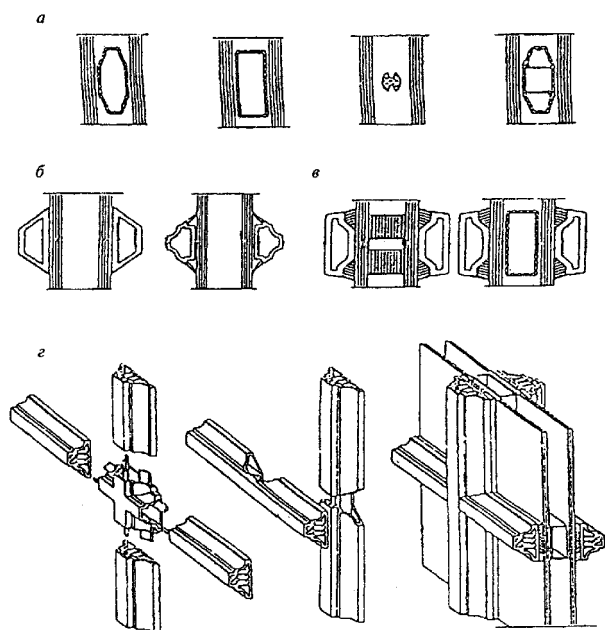
a — профили внутренней рамки стеклопакета; b — накладные декоративные раскладки; e — вариант комбинированного применения накладных раскладок и внутренней рамки стеклопакета; z — переплетные соединения раскладок
