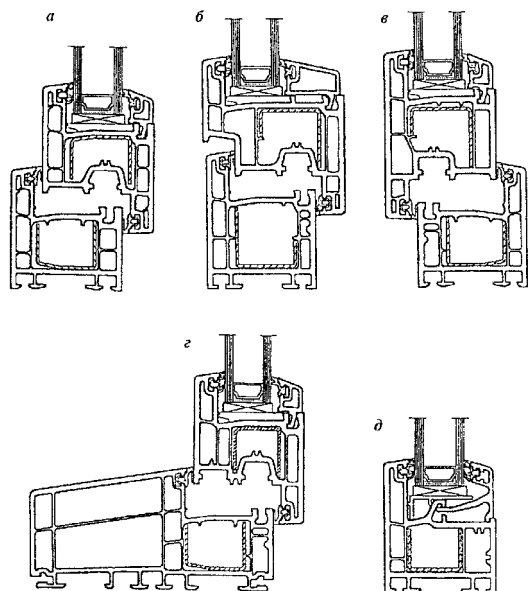
а — оконная система из трехкамерных профилей; б — оконная система с четырехкамерной створкой и трехкамерной коробкой (расположение наружных стенок створки и коробок в одной плоскости); в — оконная система из трехкамерных профилей (открывание наружу); г — оконная система из многокамерных профилей с расширенной коробкой; д — оконная система с остекленной коробкой
