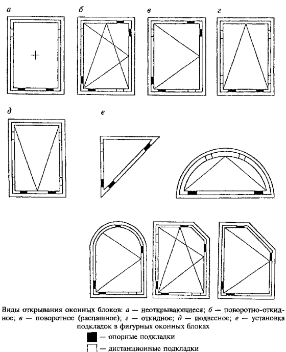
Рисунок 5 -- Схемы расположения опорных и дистанционных подкладок при монтаже стеклопакетов в зависимости от вида открывания оконных блоков
